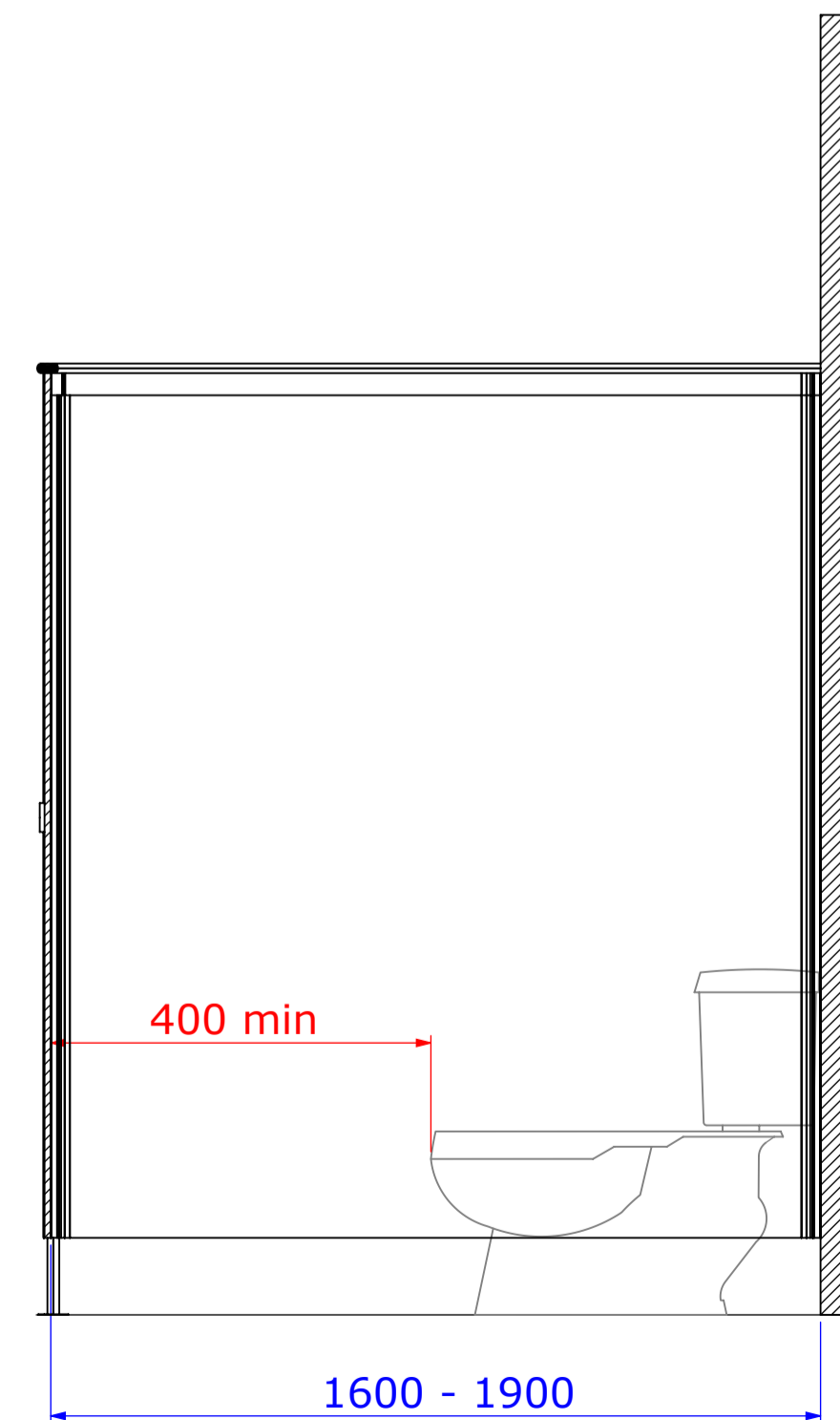
SECTION D-D
