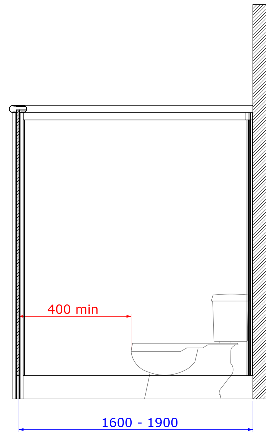
SECTION D-D
